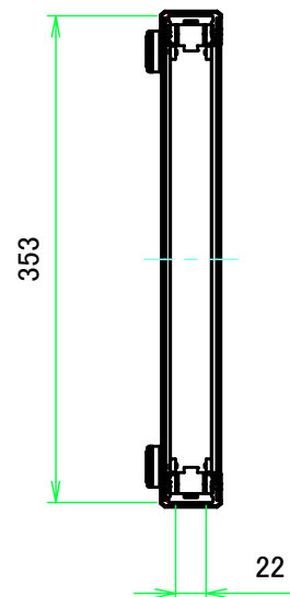
A-A (1:6)
